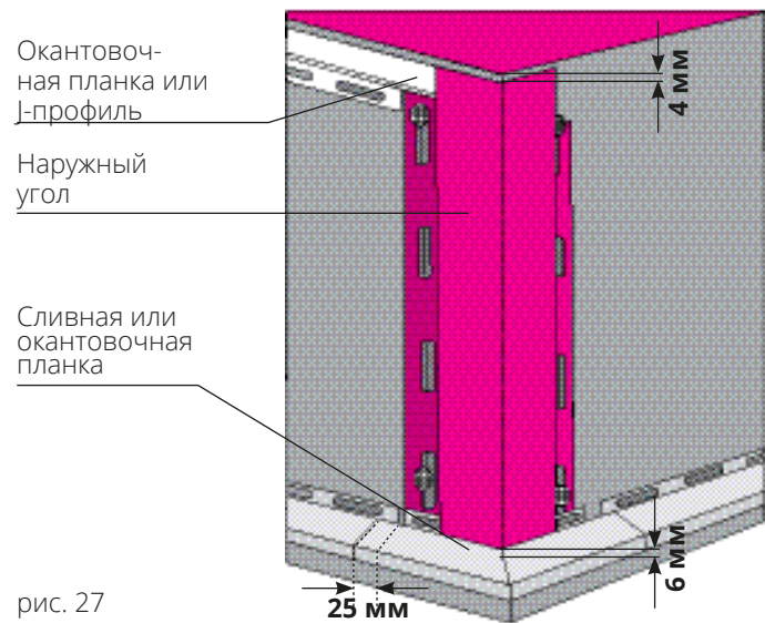
Вертикальный сайдинг
