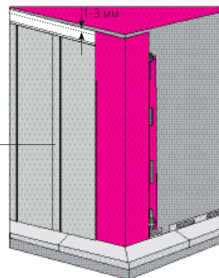
Вертикальный сайдинг
